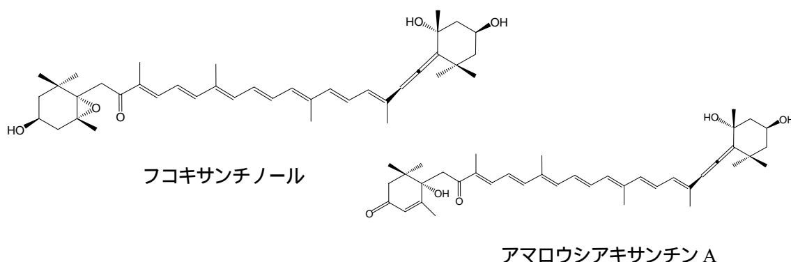
図 20 フコキサンチノールとアマロウシアキサンチン A の構造式
