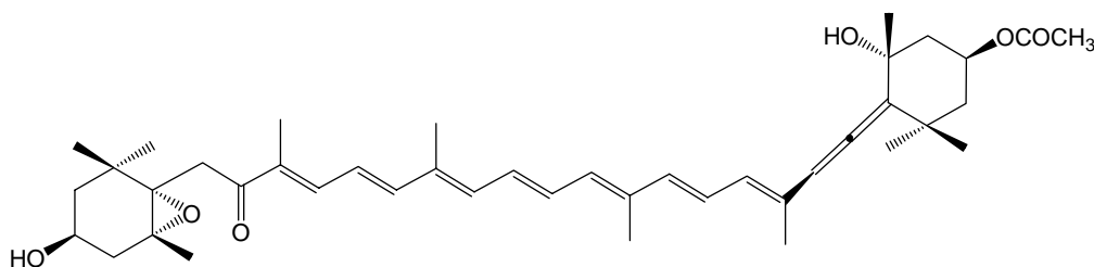
図2 フコキサンチンの構造式
