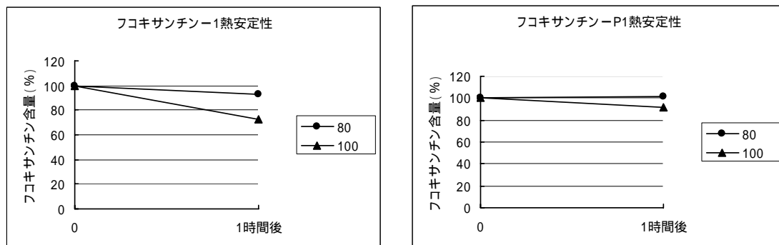
図 23 フコキサンチンの熱安定性
