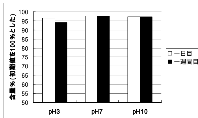
図 24 フコキサンチン-WSP0.1のpH安定性
