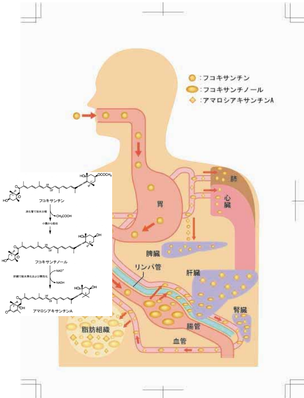
図 21 推定されたフコキサンチンの生体内代謝経路
